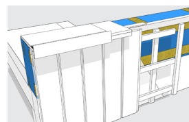
Gevelbekledingssysteem, verticale afwerking
