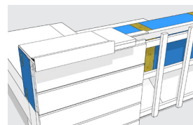
Gevelbekledingssysteem, horizontale afwerking
