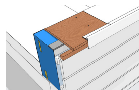
De houten dekplaat wordt vastgeschroefd aan de bovenste houtregels van het element.
