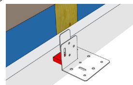
De Dakstand® G wordt vastgezet met de meegeleverde Dakstand® XL-anker.
