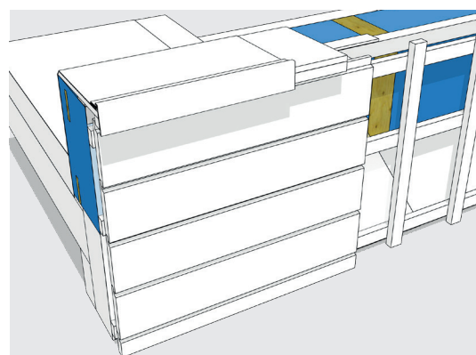
7 Aansluiting op gevelbekledingssysteem, horizontale afwerking
